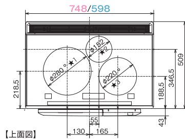
【上面図】
