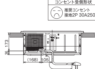
【背面図】
