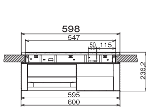
【正面図】
